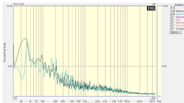
Fig. 7. Comparación del ancho de banda entre la ONYX 24-4 y la referencia
