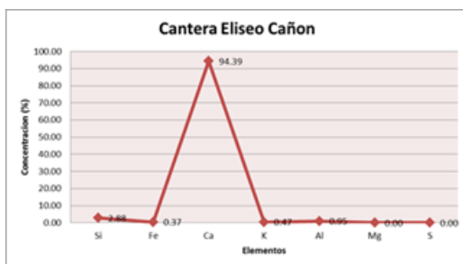
Figura 6. Composición elemental de las calizas de la cantera Eliseo Cañon
