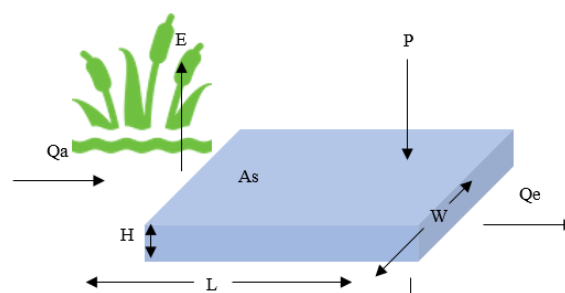
Figura 1. Esquema de un humedal artificial donde Q_a es el caudal del afluente, E es la evapotranspiración, P es la precipitación, As el área superficial, H la altura del humedal, L la longitud del humedal y W el ancho del humedal. Modificado de [2].
