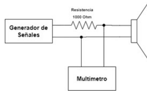
Figura 3. Diagrama de bloques para medición de curva de impedancia
