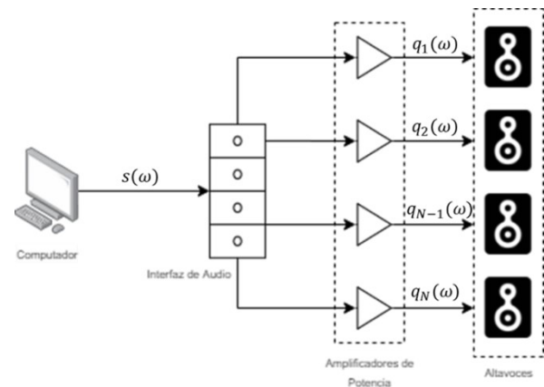
Figura 1. Configuración de N altavoces para zonas de escucha personalizadas
