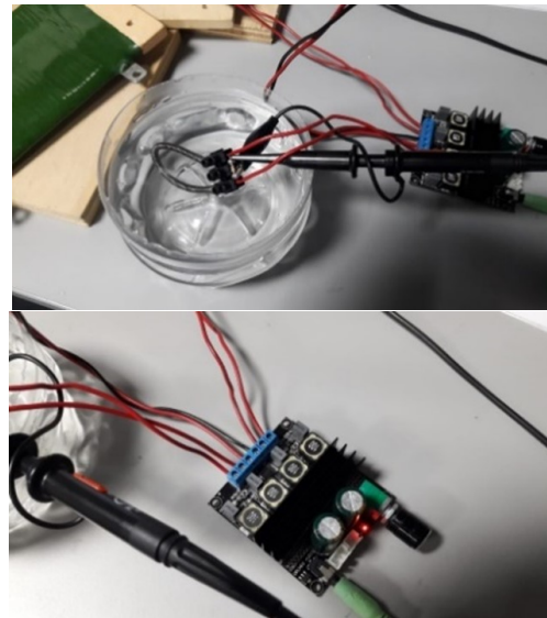
Figura 7. Montaje para la medición de distorsión armónica total
