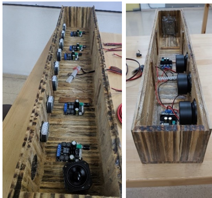
Figura 9. Cableado para arreglo de altas y bajas frecuencias
