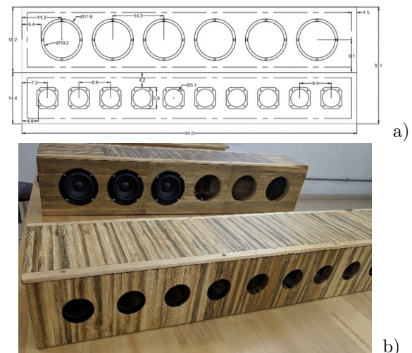
Figura 2. Etapas de construcción de las cajas acústicas. (a) Planos técnicos con dimensiones y cotas (b) Montaje parcial de altavoces en las cajas
