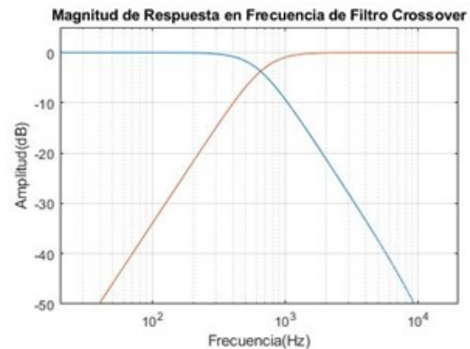
Figura 10. Magnitud de Respuesta en Frecuencia del Filtro de Cruce digital
