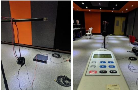
Figura 5. Configuración utilizada para la medición de respuesta en frecuencia
