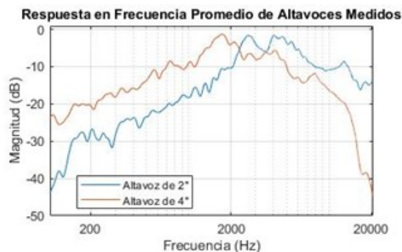
Figura 6. Respuesta en Frecuencia promedio para altavoces de 2" y 4" respectivamente
