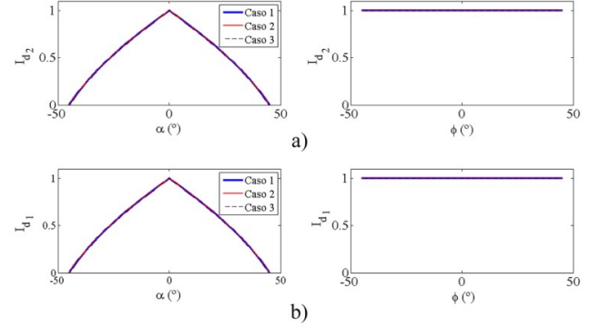
Figura 14. Evaluación de I_{d2} e I_{d1} para remolques 1 y 2 con articulación esférica, variando L_1 y L_2
