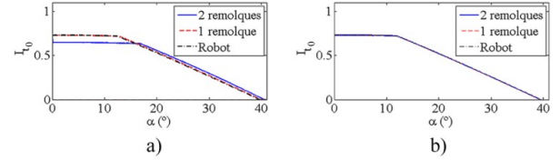
Figura 6. Evaluación de I_{t0} con diferente cantidad de cuerpos
