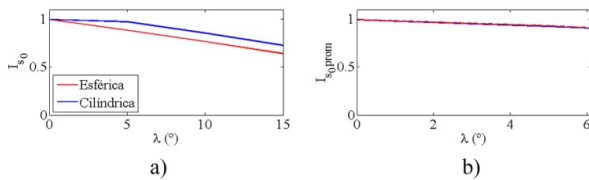
Figura 5. Evaluación de I_{s0} con diferente articulación
