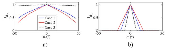
Figura 15. Evaluación de I_{d2} e I_{d1} para remolques 1 y 2 con articulación cilíndrica, variando L_1 y L_2
