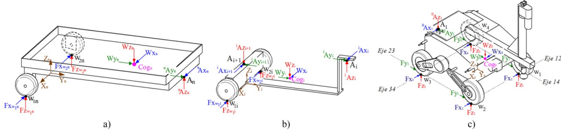
Figura 2. Nomenclatura y fuerzas de reacción en el robot Lázaro y los remolques acoplados
