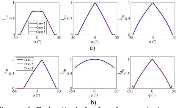
Figura 12. Evaluación de I_{t0} , I_{s0} e I_{d0} para el robot con articulación cilíndrica, variando L_1 y L_2
