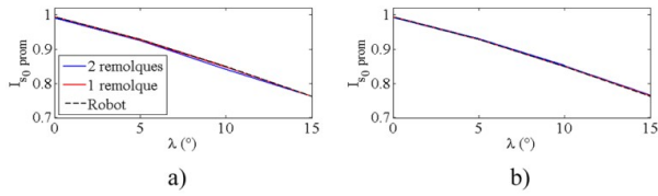
Figura 8. Evaluación de I_{s_0} con diferente cantidad de cuerpos (Trayectoria circular)
