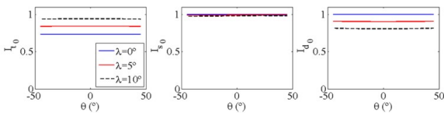
Figura 17. Efecto de la variación de \theta en I_{t_0} , I_{s_0} e I_{d_0}
