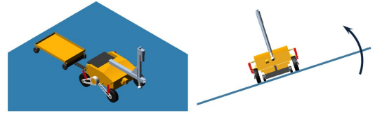
Figura 3. Prueba realizada en ADAMS para verificar la navegabilidad del robot con remolques
