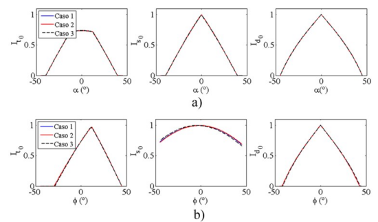
Figura 11. Evaluación de I_{t_0} , I_{s_0} e I_{d_0} para el robot con articulación esférica, variando L_1 y L_2
