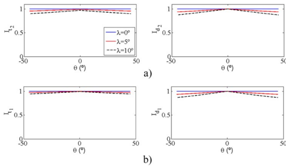
Figura 19. Evaluación de I_{ti} e I_{di} para remolques con articulación esférica, variando \theta en solo en remolques 1 y 2
