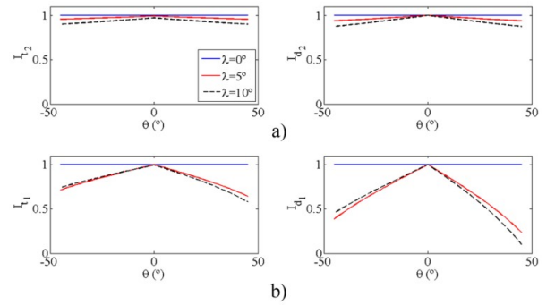
Figura 18. Evaluación de I_{t_i} e I_{d_i} para remolques con articulación esférica, variando \theta en solo en el remoque 2
