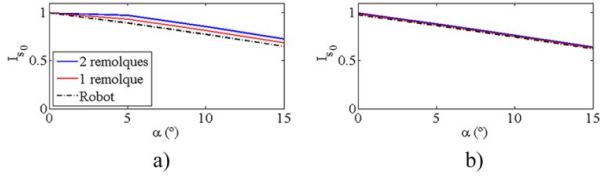
Figura 7. Evaluación de I_{s_0} con diferente cantidad de cuerpos (Trayectoria recta)
