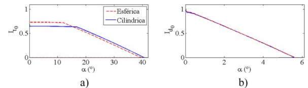
Figura 4. Resultados de simulación ( I_{t_0} e I_{d_0} ) con diferente articulación
