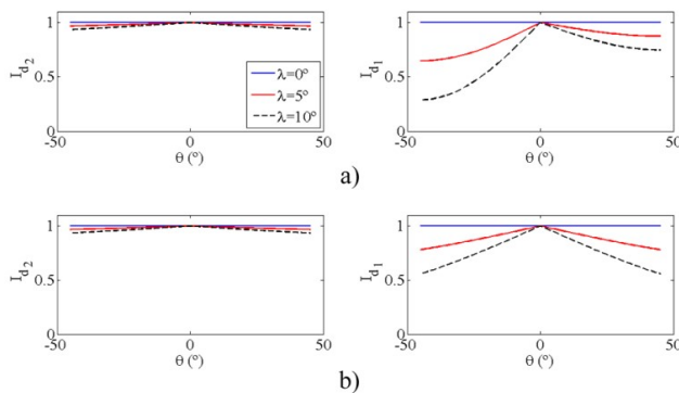
Figura 20. Evaluación de I_{di} para remolques con articulación cilíndrica, variando \theta en: a) remolque 2; b) remolques 1 y 2
