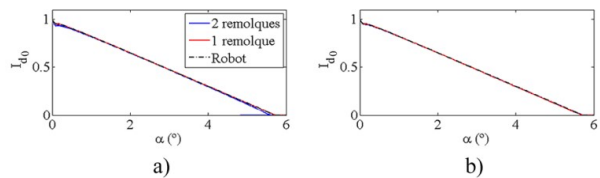
Figura 9. Evaluación de I_{d_0} con diferente cantidad de cuerpos
